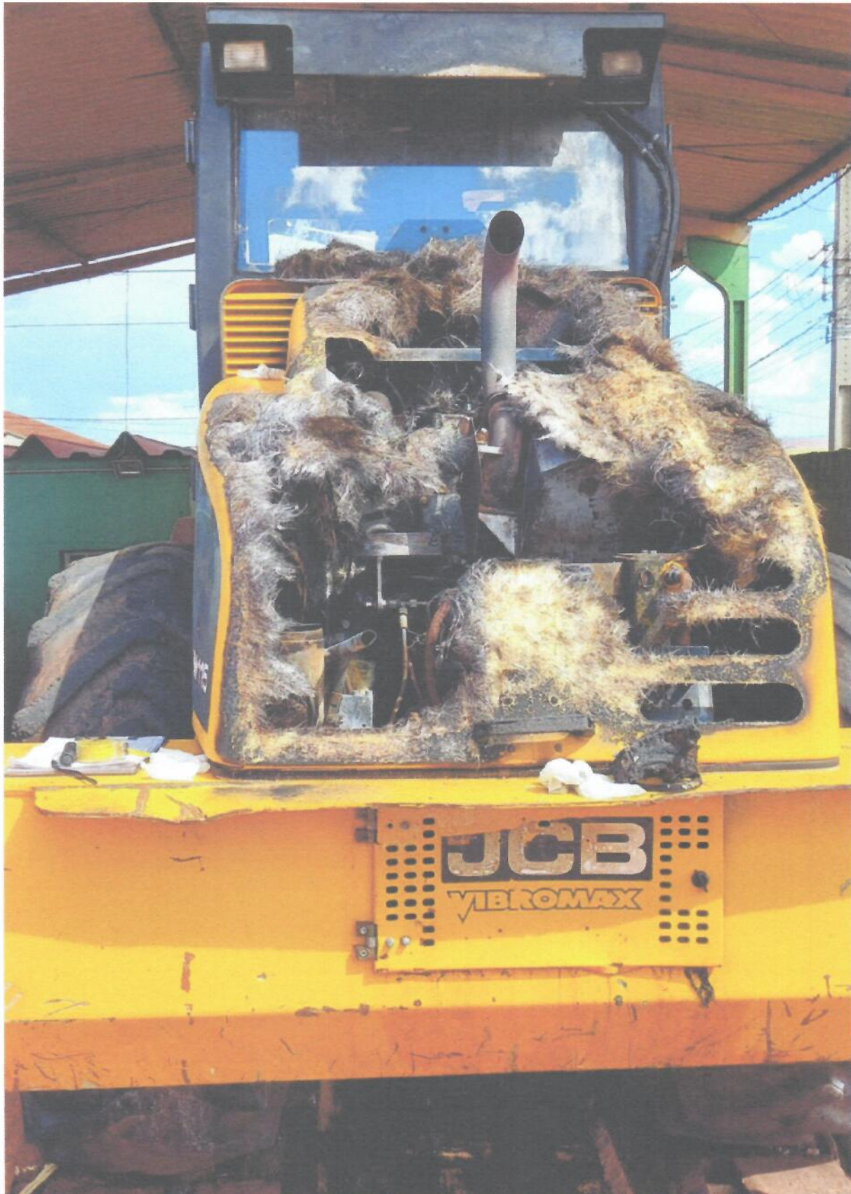
Imagem 05. Região posterior do equipamento periciado (região afetada pelo fogo).
